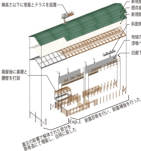
旧音楽体育室 (カフェレストラン)：廊下との間の界壁に用いられていた柱・建具を手前に移設し、天井木ルーバーは既存の高さに合わせた
