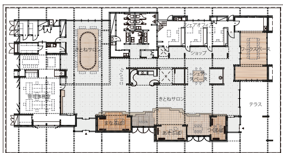
平面図 S=1/600
